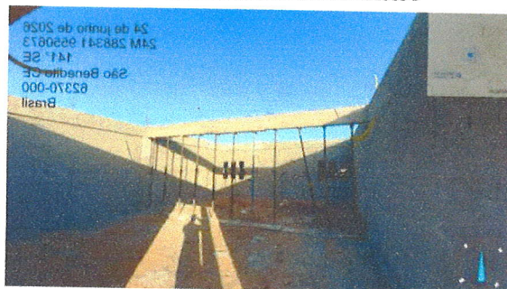
FUNDAÇÕES, ESTRUTURA E ALVENARIA BLOCO B
